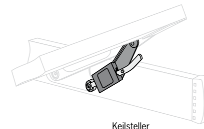
Keilsteller
